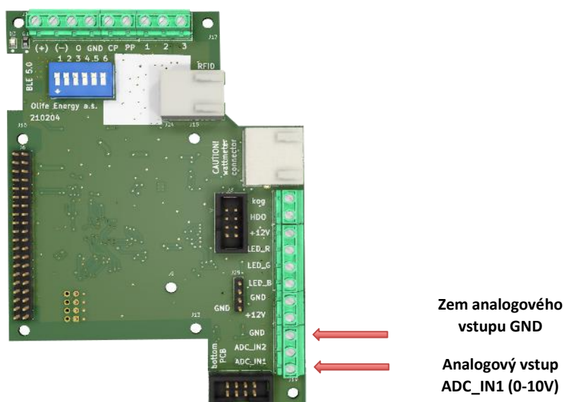
Obrázek 16: Zapojení řídicího vodiče
